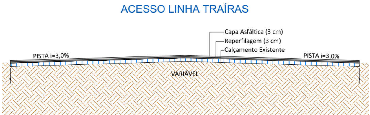
SEÇÃO TIPO ESCALA: 1 : 50
