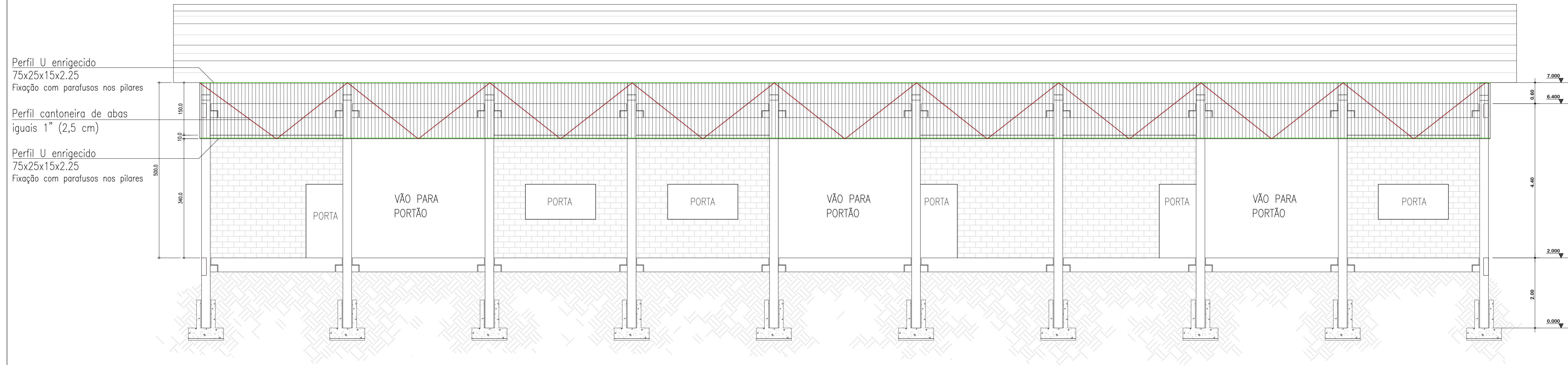
↑ Detalhe: Fechamento Lateral Escala: 1:50 → x
