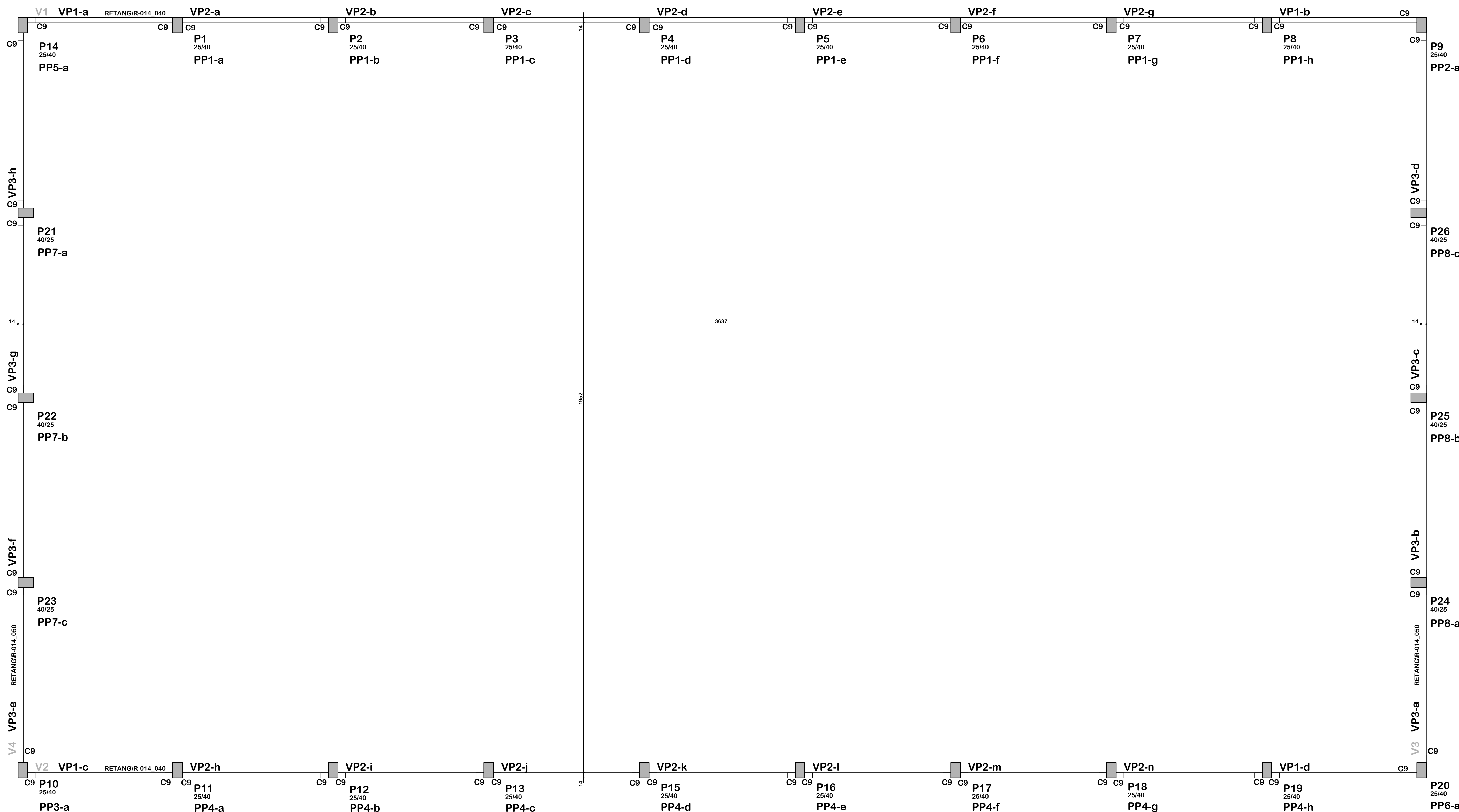
Planta de formas: Baldrame Escala: 1:50
