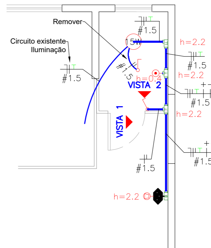
PLANTA BAIXA - Sanitário PCD ESC.:1/50
