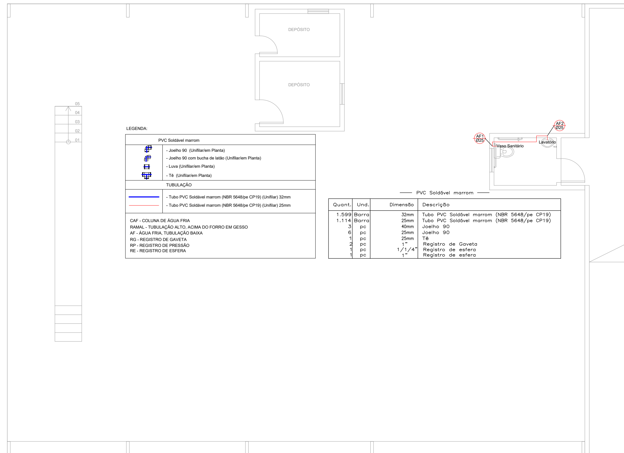
PLANTA BAIXA BLOCO 3 - HIDRÁULICO ESC.:1/75
