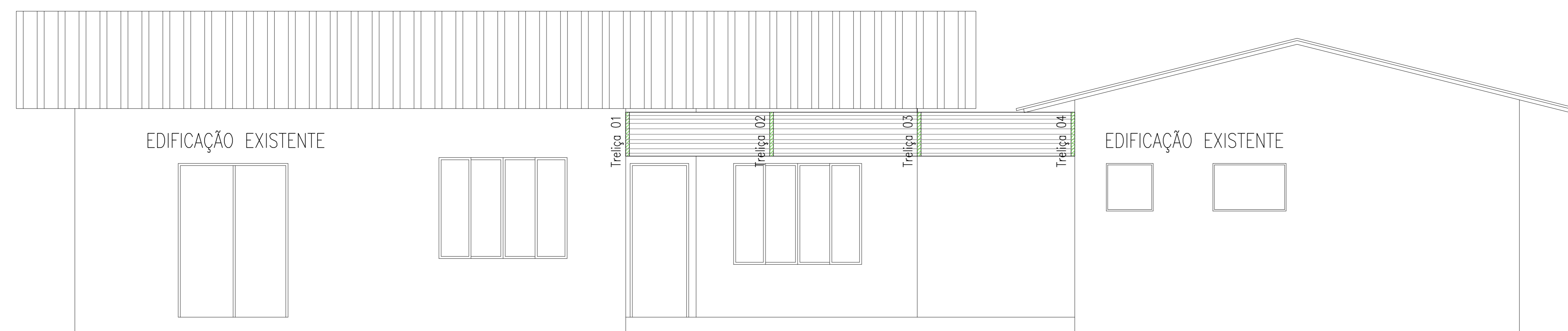
Y VISTA FRONTAL – COBERTURA METÁLICA Escala 1:50 X
