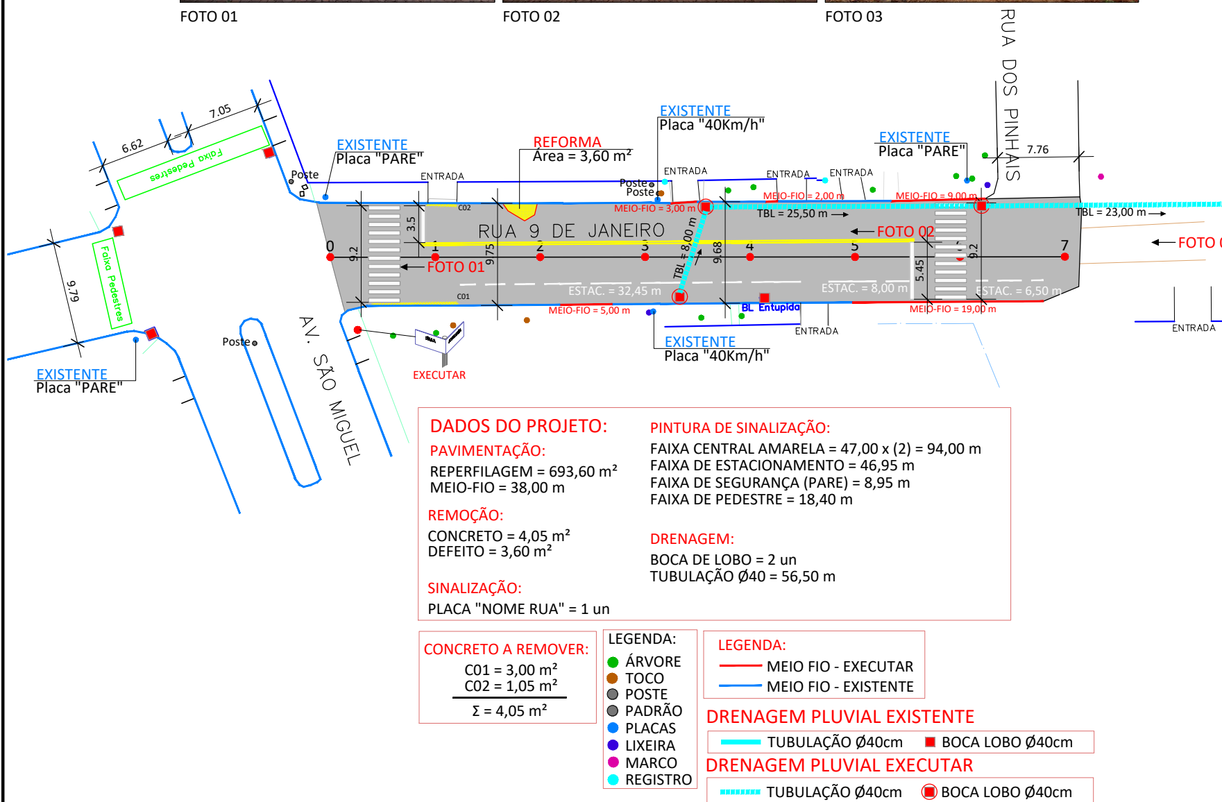
PLANIALTIMÉTRICO ESC.: 1:500
