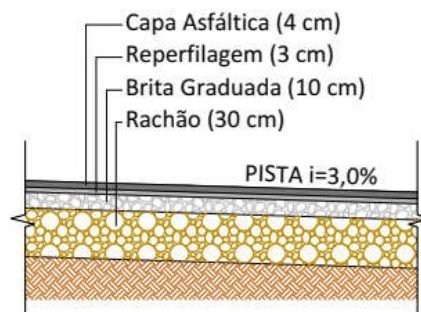
DETALHE REMENDO ESCALA: 1 : 50
