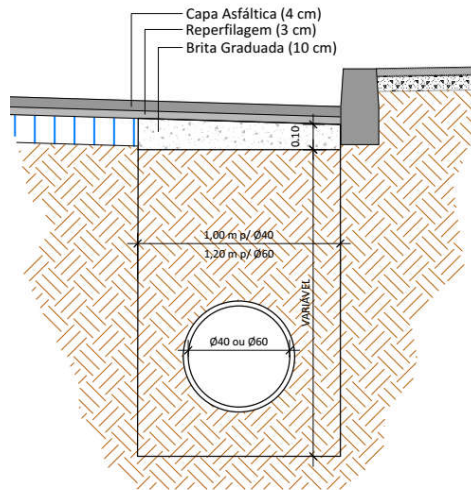
DETALHE REMENDO ESCALA: 1 : 25
