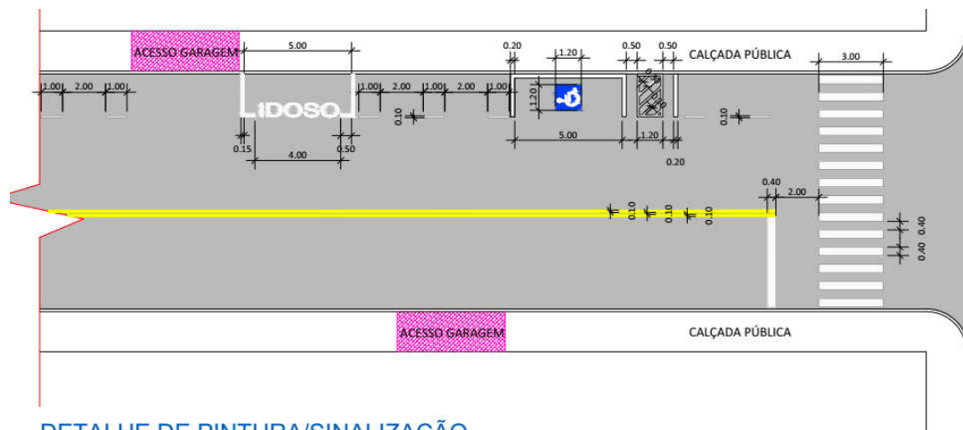
DETALHE DE PINTURA/SINALIZAÇÃO ESC.: 1:150
