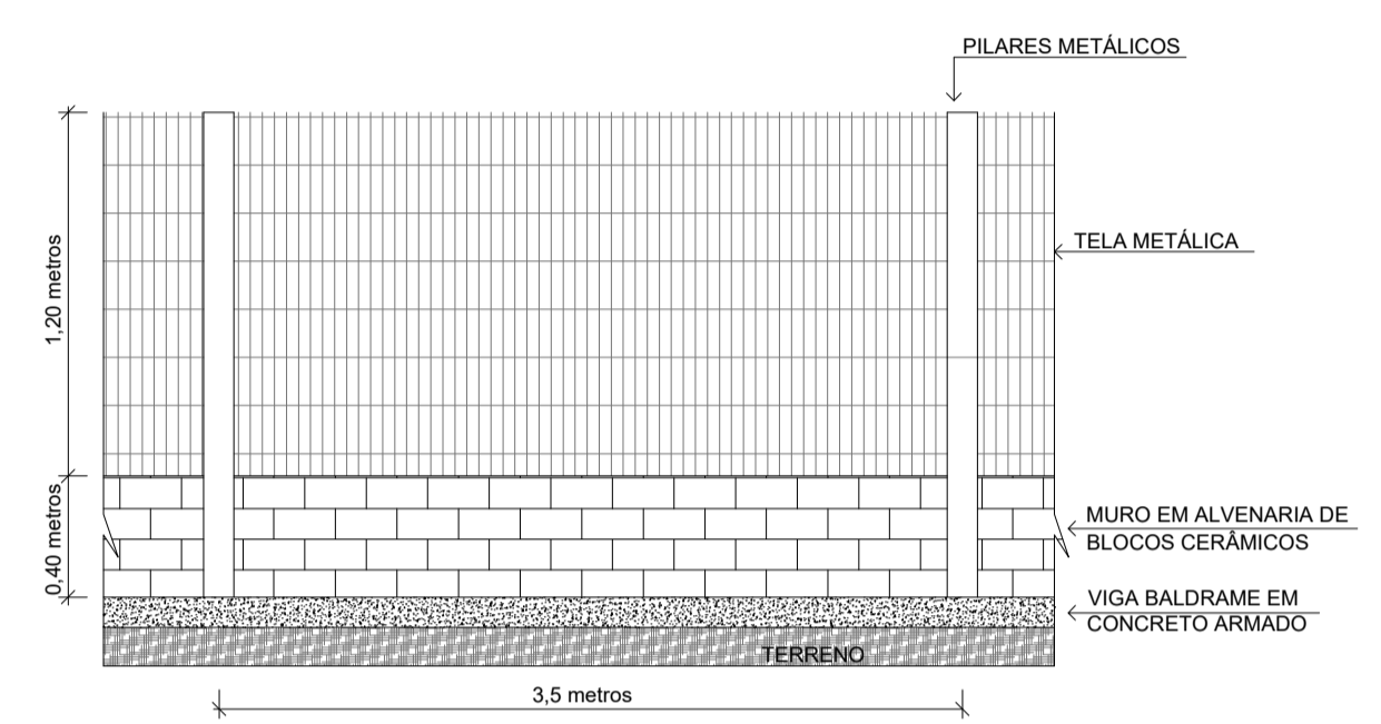
DETALHE MURO ESC: 1/50
